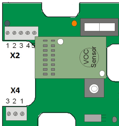
Klemmenansicht innen
